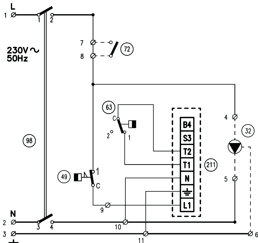
рис. 7 - Принципиальная электрическая схема EL-DB N 32 ч 78
