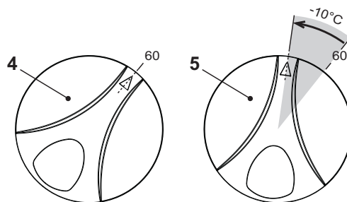
рис. 3 - Регулирование температуры модели EL-DB N 95
