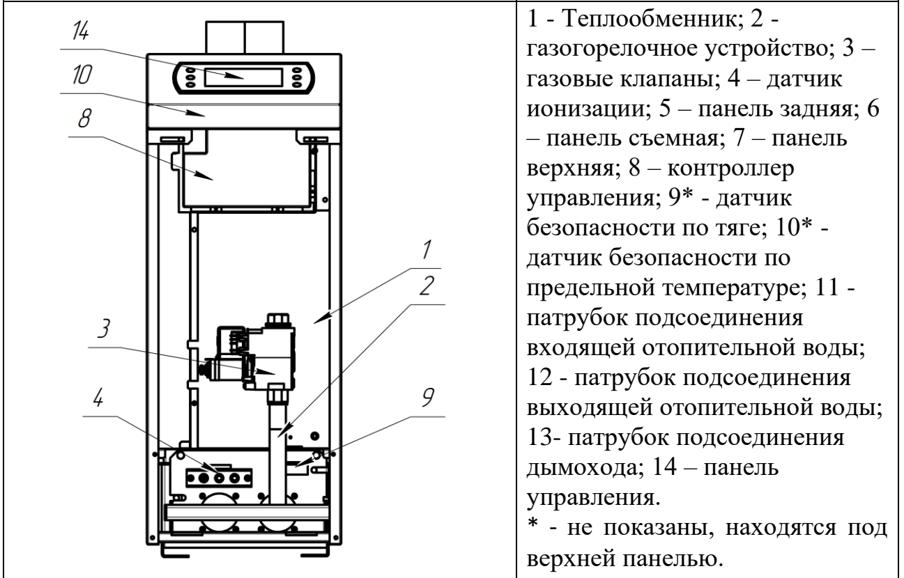
Рисунок 1 – конструкция котла AXIS SMART
