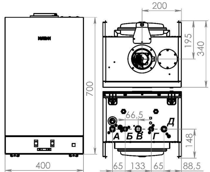
Рис. 12. Габаритные и присоединительные размеры.
