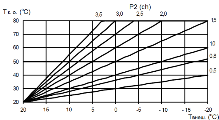
Рис. 3 График зависимости температуры в контуре отопления от внешней температуры при комнатной температуре 20 °С
