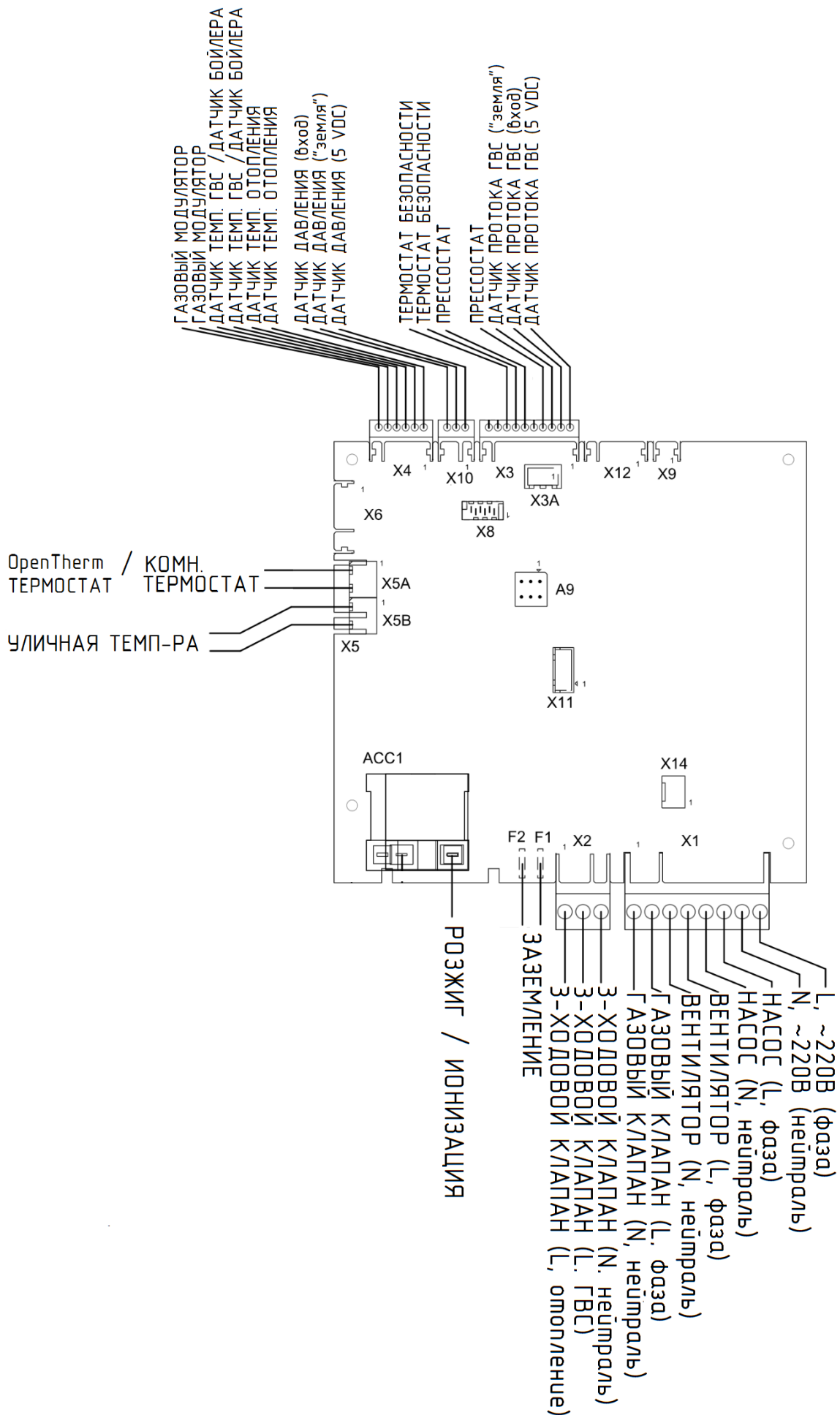
Рис. 14. Электрическая схема
